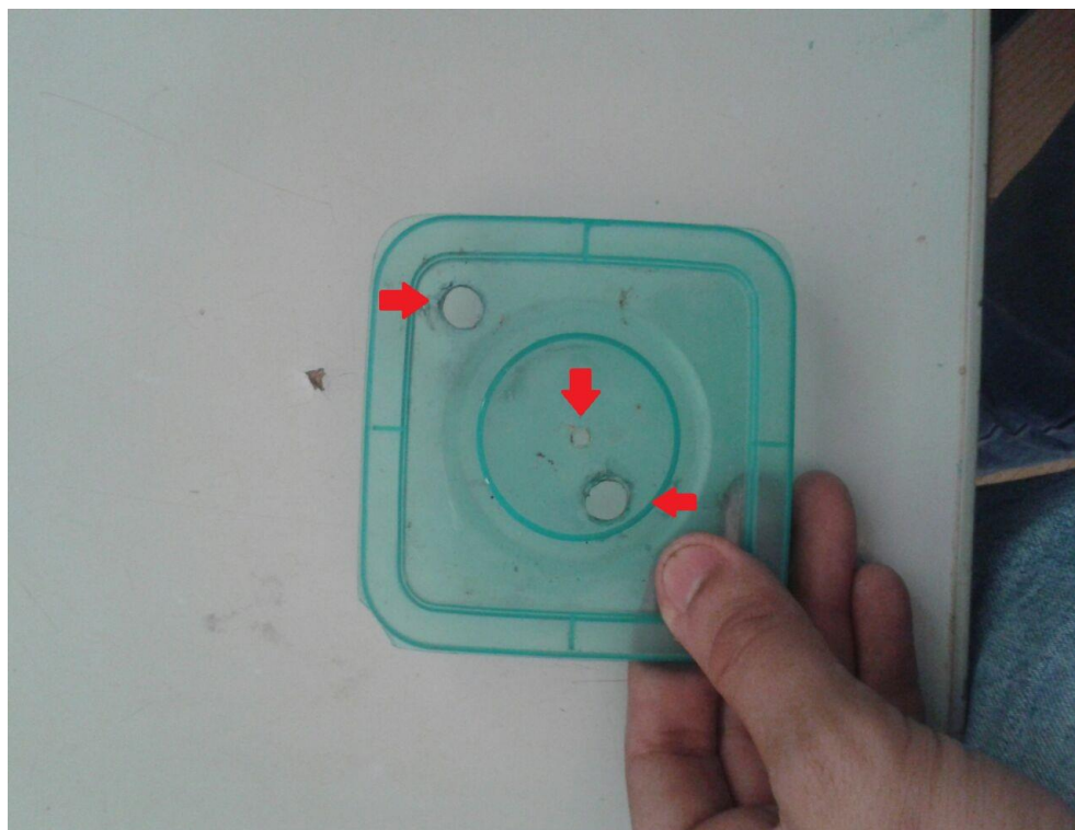
FIGURA 1 – Tampa da cuba eletrolítica
